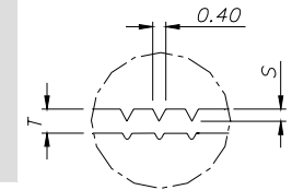
SECTION D-D
